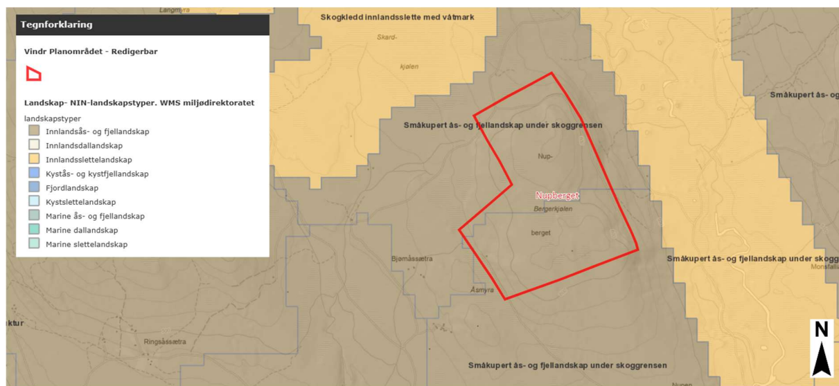
Figur 5.4: NiN landskapstyper.
